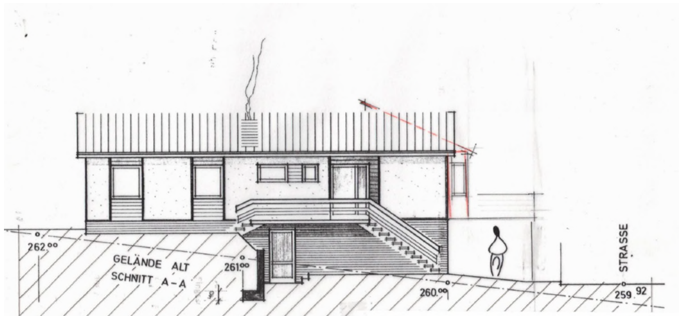
Ansicht Ost
