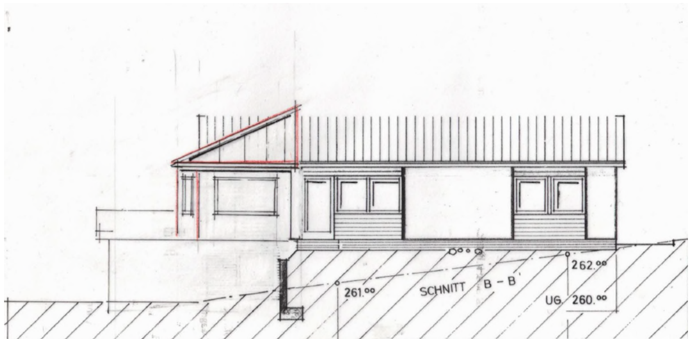
Ansicht West
